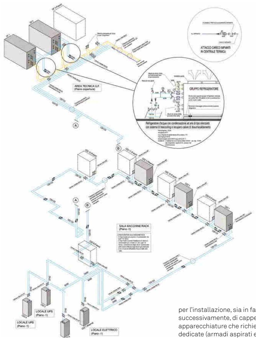
Schema assonometrico dell'impianto di climatizzazione del Data Center
