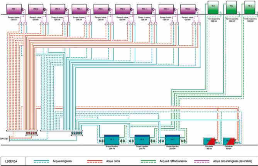
Produzione termofrigorifera mensile Schema funzionale semplificato della produzione termofrigorifera
