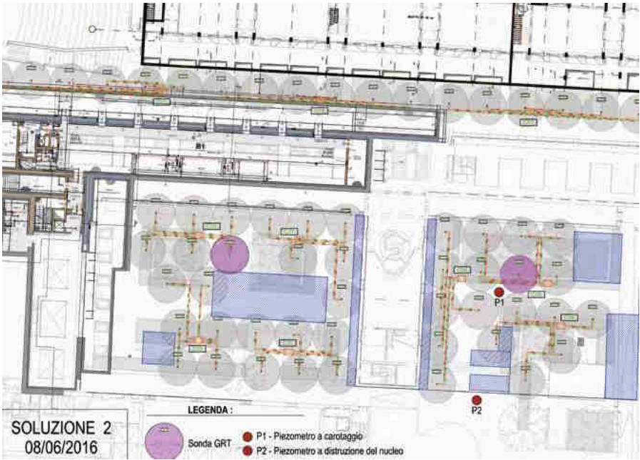
Posizione delle sonde geotermiche e dei piezometri per il monitoraggio del campo sonde
