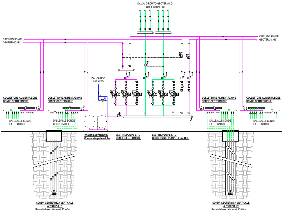
Schema funzionale della sottocentrale tecnologica tipo
